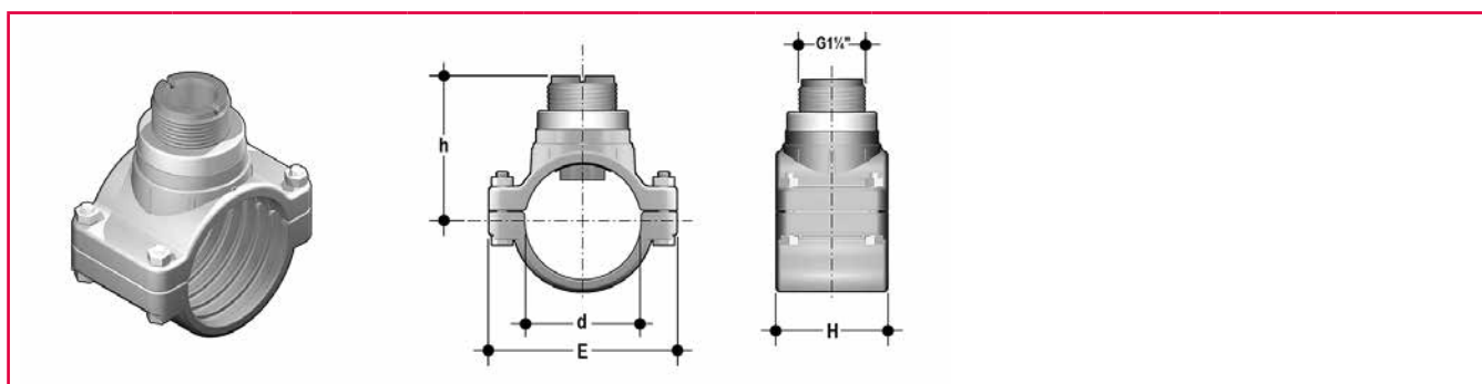
Трубные зажимы ASTM
