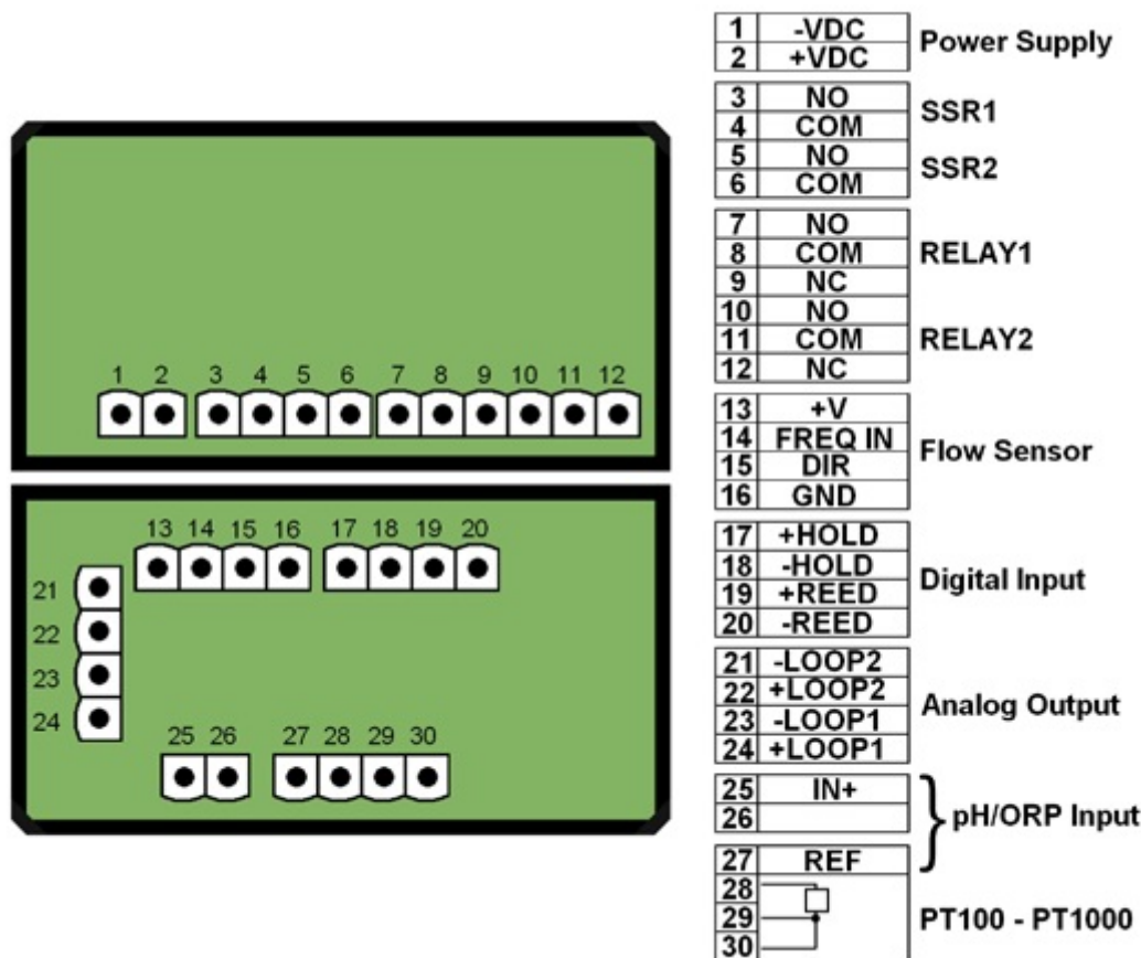
мониторы pH/овп и расхода M9.08
